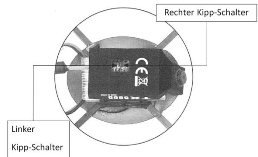
Kanal 4 Schalterposition
